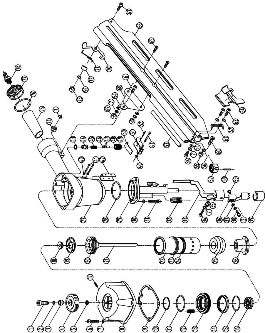
Рисунок 1 – Схема пневматического гвоздезабивного пистолета FN-2190 KIRK
