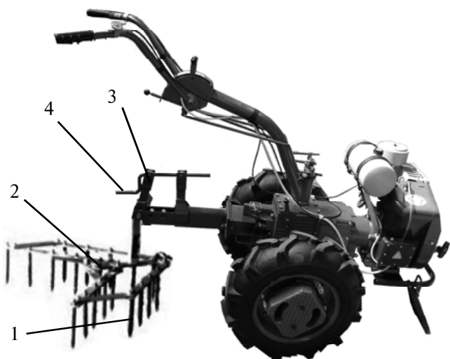
1 - борона, 2 - рукоятка бороны, 3 - универсальное устройство поворотного механизма, 4 - рукоятка универсального устройства поворотного механизма
