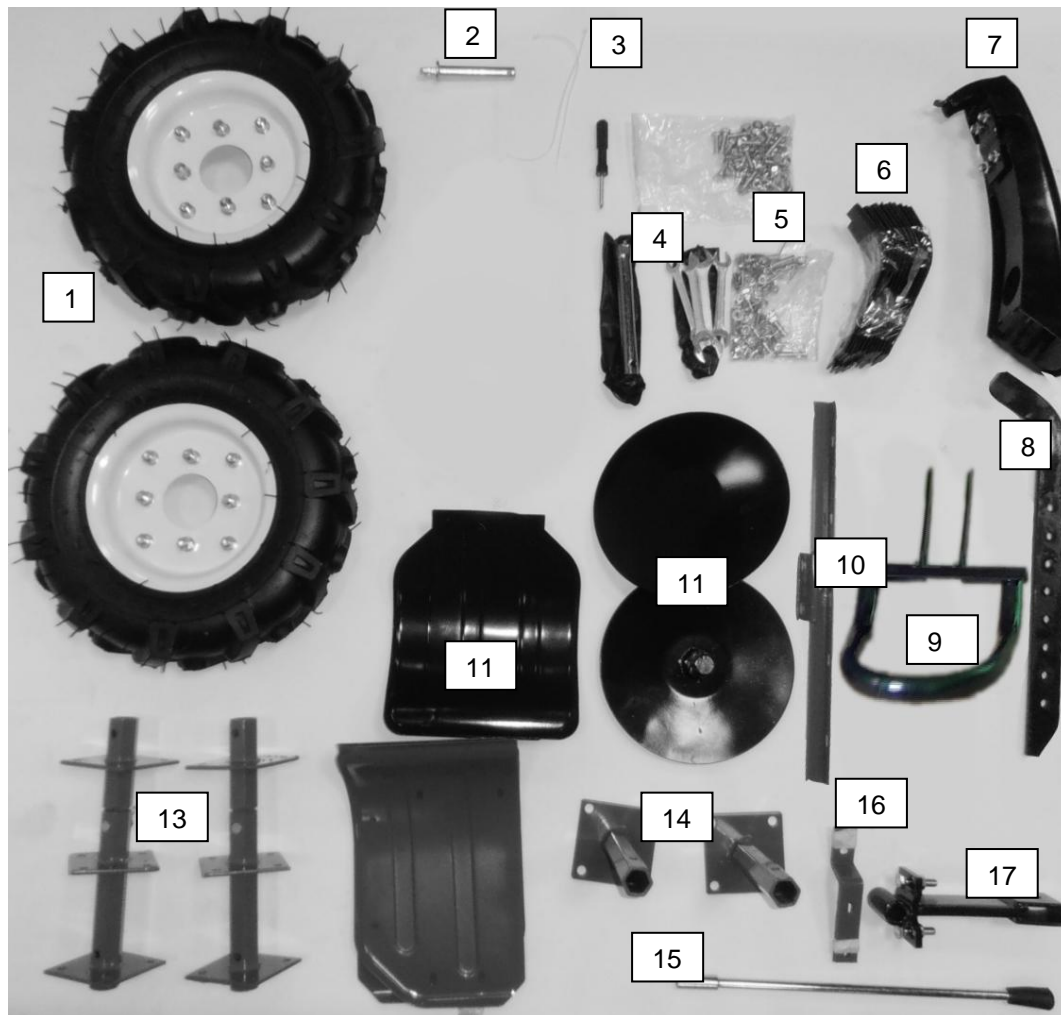
Рис. 2. Комплект поставки.
