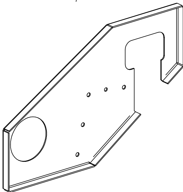
ТН214.00.005 Кронштейн
