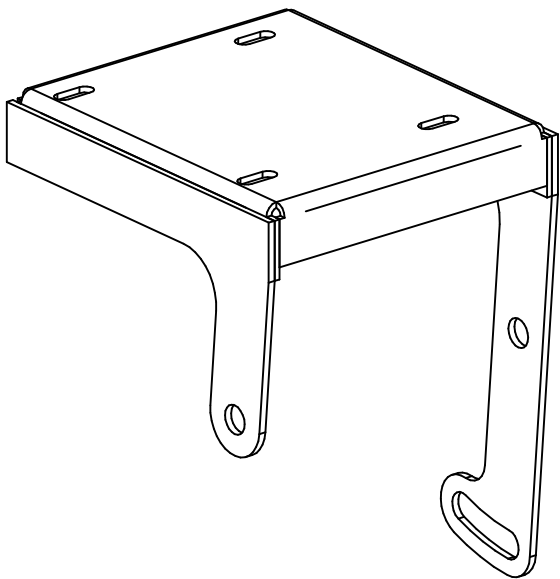
ТН214.07.000 Кронштейн
