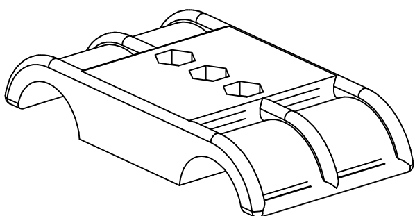
ТН107.00.00.009 Прижим
