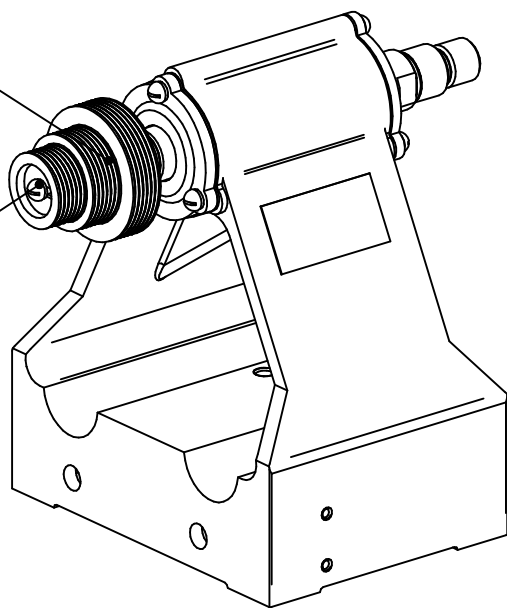
ТН107.00.00.009 Прижим
