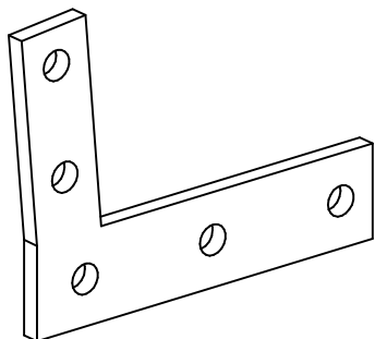
ТН214.00.007 Проставка
