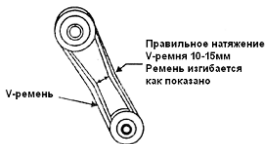
Рис. 2 Натяжение V-ремня
