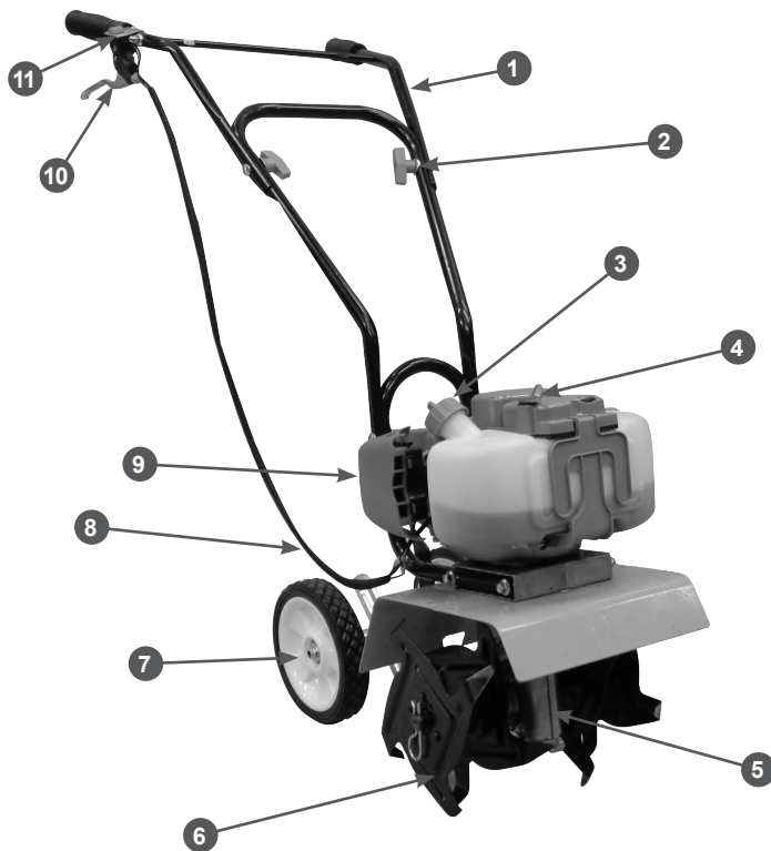
Рис. 1 Основные узлы и органы управления
