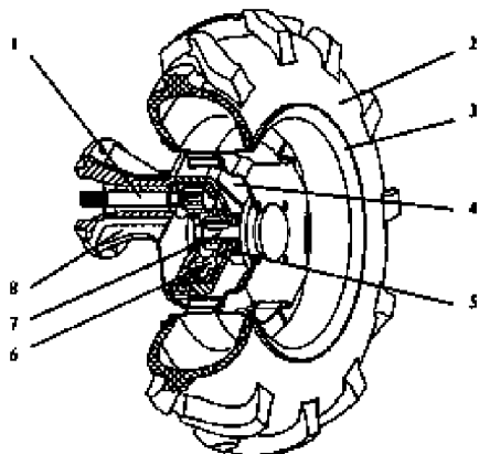
Рисунок 1.12 - Конечная передача
