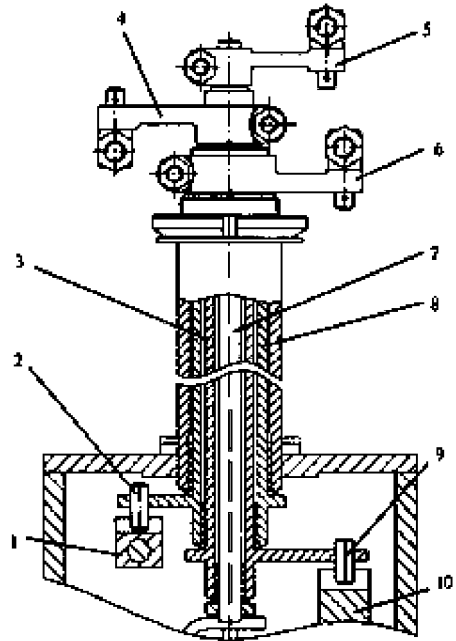
1 - поводок, 2 - штифт, 3 - вал режимов, 4 - рычаг режимов, 5 - рычаг блокировки дифференциала, 6 - рычаг передач, 7 - ват блокировки, 8 - вал передач, 9 - штифт, 10 - поводок
