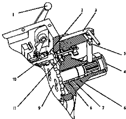
Рисунок 1.13 - Сцепка ВОМ
