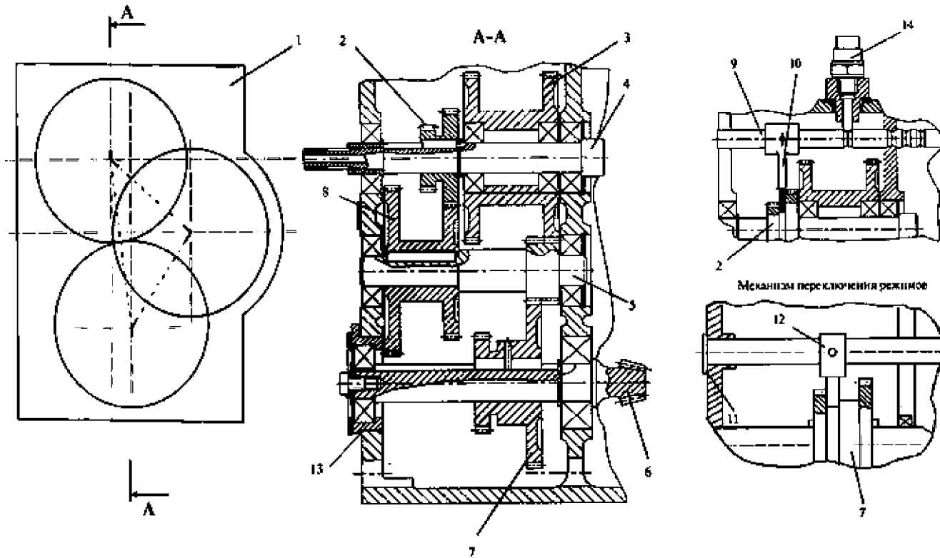
1-корпус трансмиссии, 2-блок шестерня передач, 3 –блок шестерня реверса, 4 –вал первичный, 5 –промежуточный вал шестерня,6 –вал вторичный, 7 –блок -шестерня режимов,8- блок-шестерня, 9 –скалка передач, 10-вилка, 11 – скалка режимов, 12 –вилка, 13 –стакан, 14 –механизм блокировки запуска двигателя. Рисунок 1.10 – Схема коробки передач
