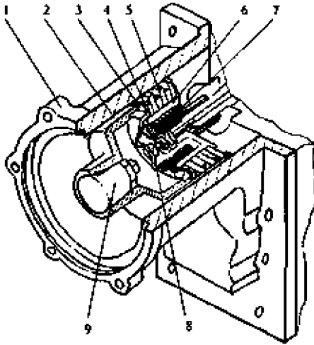
1 - корпус, 2 - полумуфта ведущая, 3 - диск нажимной, 4 - диск ведущий с накладками, 5 - диск ведомый, 6 - полумуфта ведомая, 7 - блок пружинный, 8 - толкатель, 9 - вал двигателя
