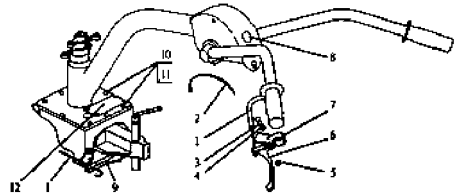
Рисунок 1.8 - Управление сцеплением 1 - тяга сцепления, 2 - хомут, 3 - болт, 4 - шайба, 5 - гайка, 6 - рычаг управления сцеплением, 7 - кронштейн, 8 - сигнальная лампочка контроля давления масла, 9 - рычаг сцепления, 10 - болт, 11 - шайба, 12 - табличка с заводским номером моторного блока.
